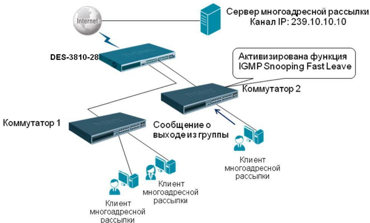
Рис. 8.7. Схема сети для настройки функции IGMP Snooping Fast Leave
