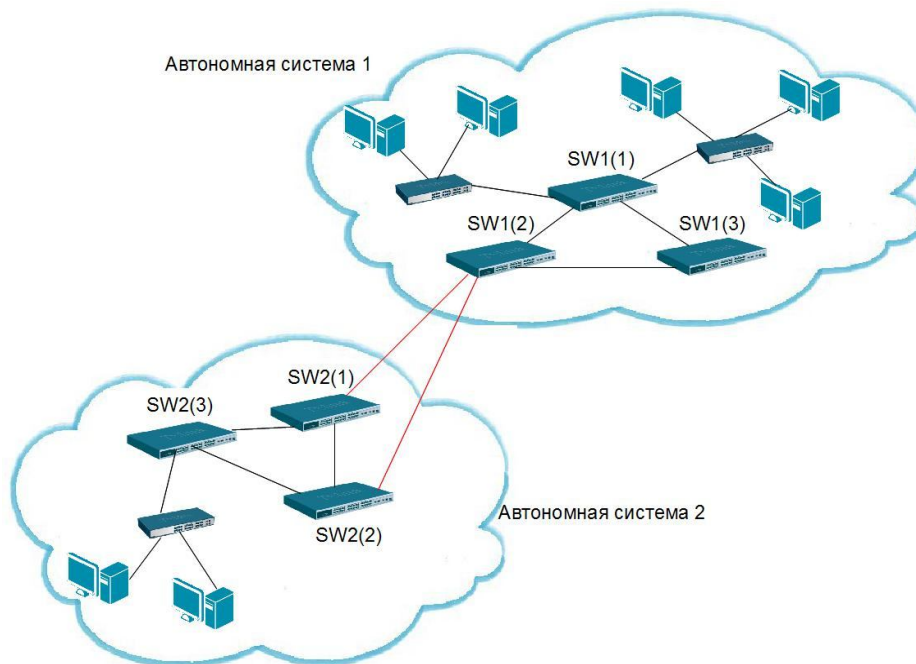
Рис. 5.44. Автономные системы
