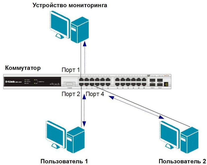
Рис. 9.16. Функция Port Mirroring
