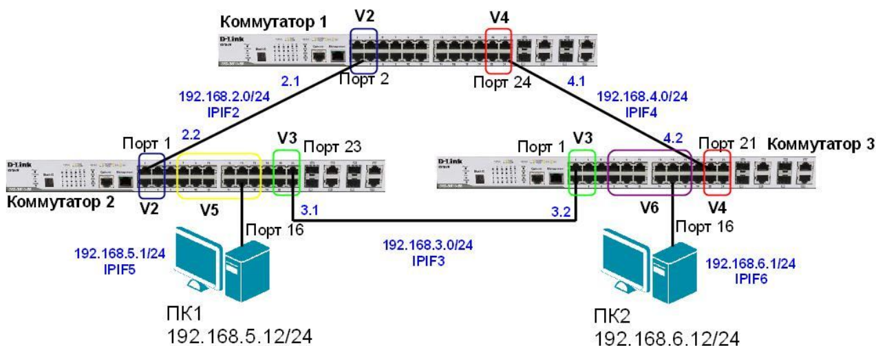
Рис. 5.57. Схема сети для настройки протокола RIPv2
