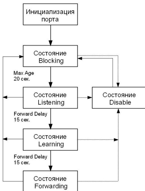
Рис. 4.4. Состояния портов при работе STP
