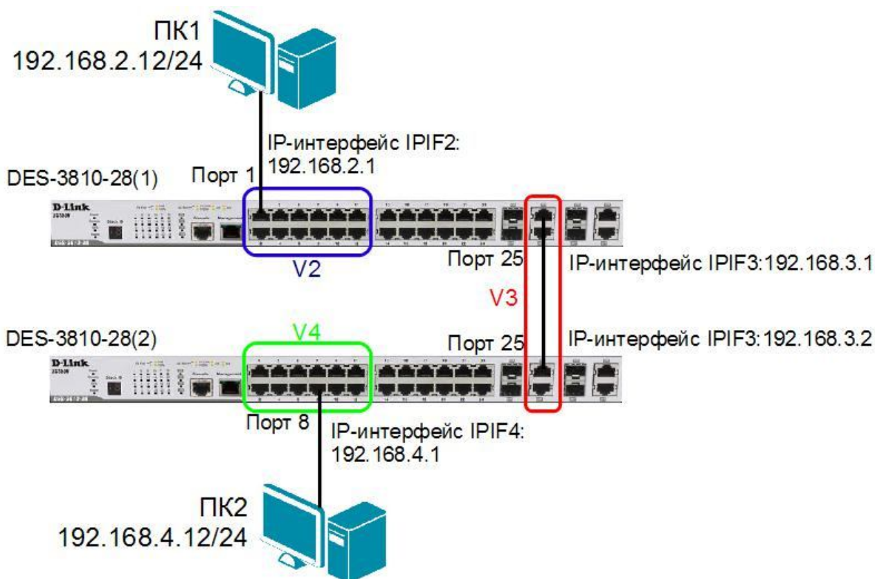
Рис. 5.42. Схема сети со статической IPv4-маршрутизацией
