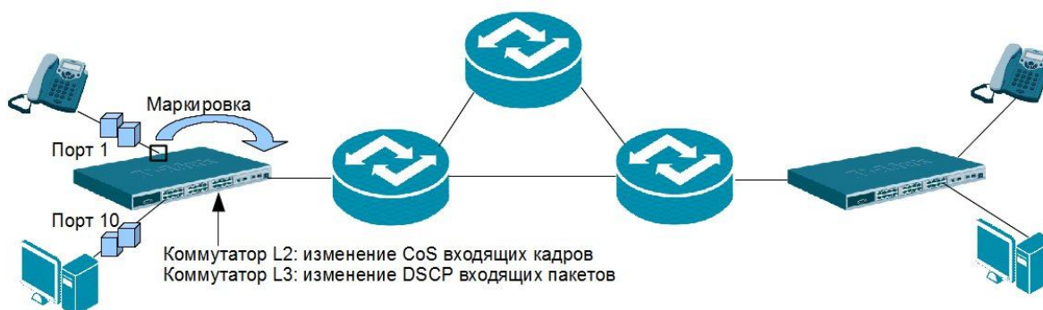
Рис. 6.3. Маркировка пакетов
