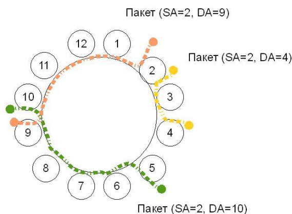
Рис. 9.1. Пример выбора оптимального пути передачи пакета в кольцевом стеке
