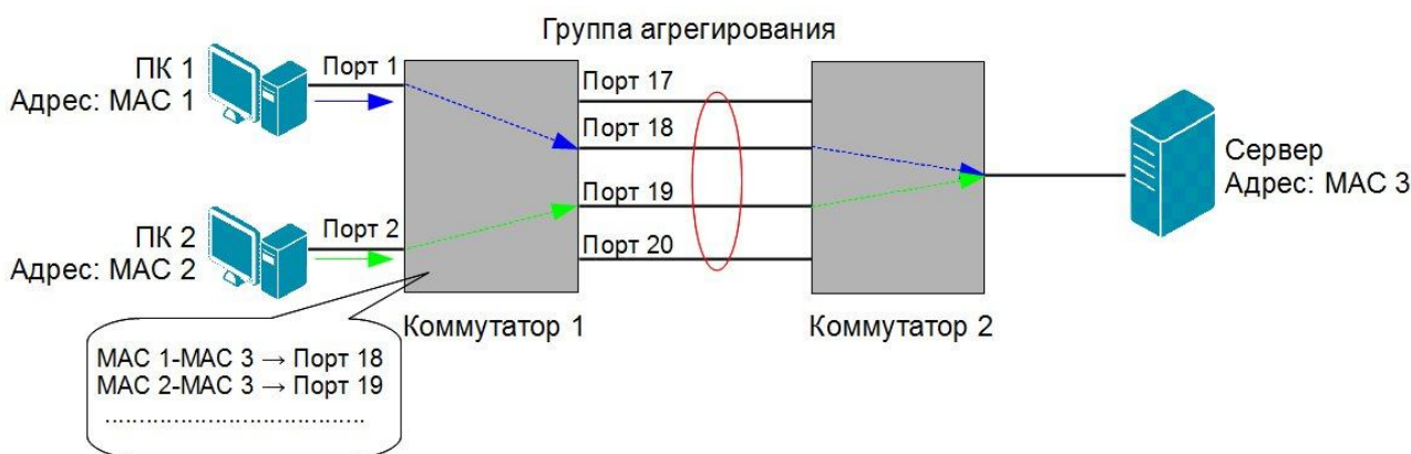
Рис. 4.28. Распределение потоков данных по каналам агрегированной линии связи для алгоритма mac_source_dest
