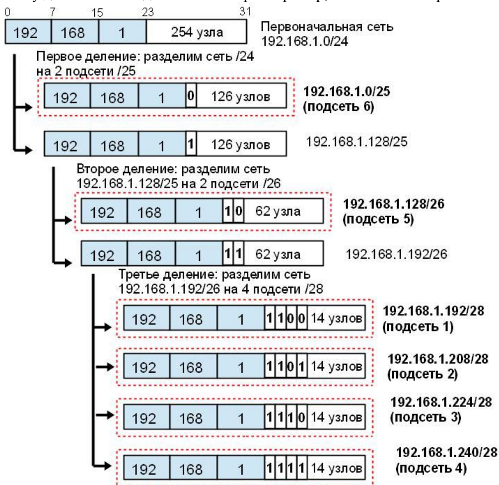
Рис. 5.17. Пример разбиения сети 192.168.1.0/24 на подсети при помощи VLSM
