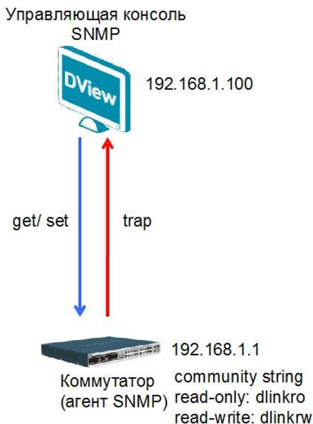
Рис. 9.14. Схема сети
