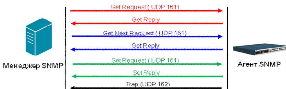
Рис. 9.13. Типы сообщения протокола SNMP
