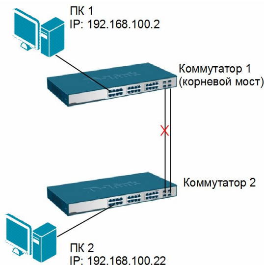
Рис. 4.6. Схема сети для настройки STP
