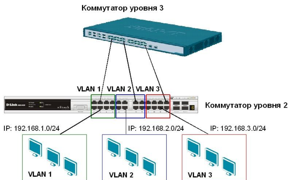
Рис. 3.4. Объединение VLAN с помощью маршрутизирующего устройства
