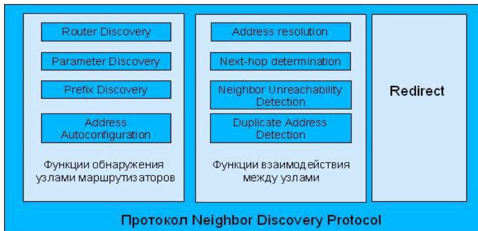
Рис. 5.34. Функции, выполняемые протоколом NDP
