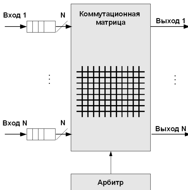
Рис. 1.18. Архитектура на основе коммутационной матрицы с входными очередями
