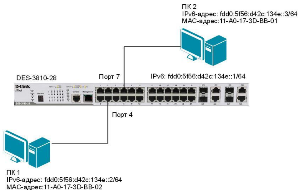
Рис. 5.37. Схема сети для проверки создания NDP-таблицы
