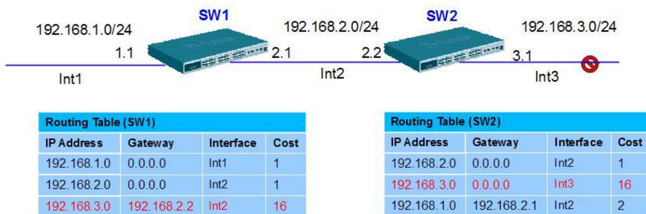
Рис. 5.48. Механизм ограничения максимального числа переходов
