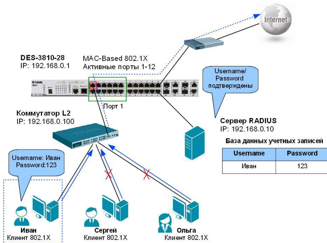
Рис. 7.17. Аутентификация 802.1X на основе MAC-адресов
