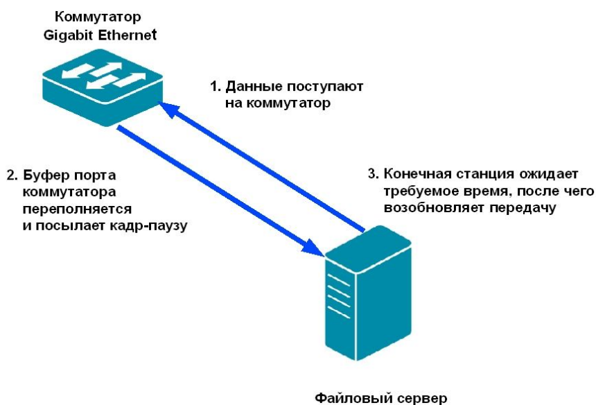
Рис. 1.22. Последовательность управления потоком IEEE 802.3x
