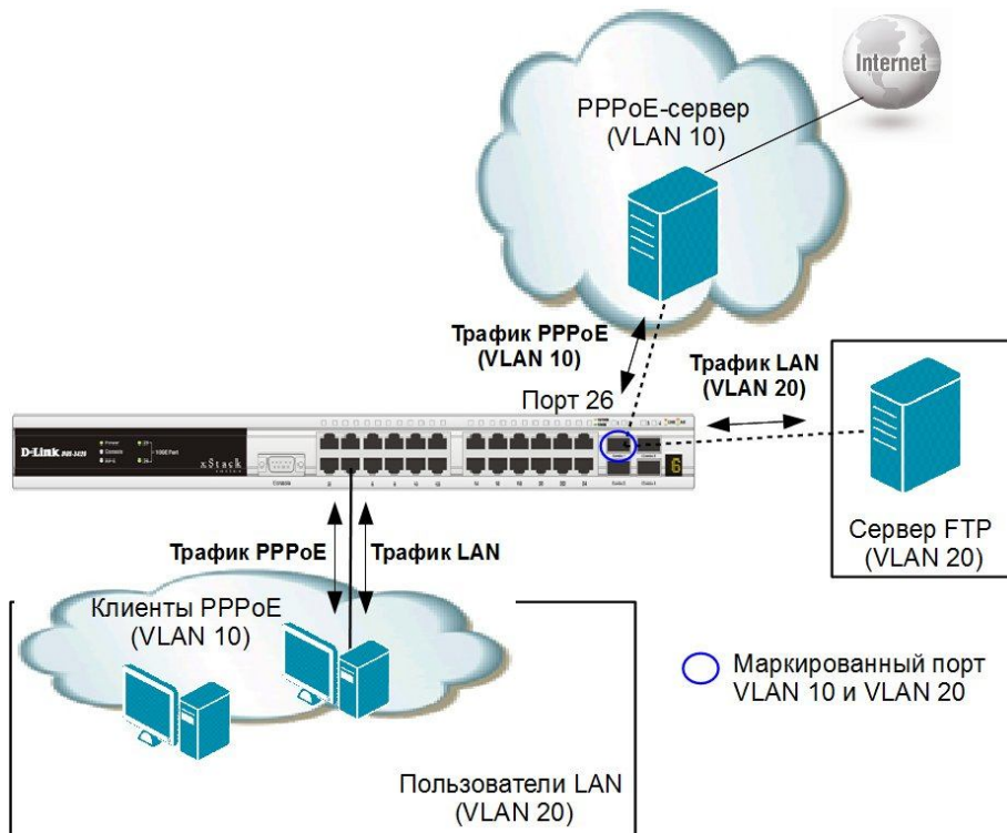
Рис. 3.23. Схема сети с IEEE 802.1v VLAN
