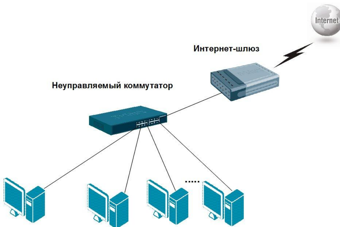
Рис. 10.1. Неуправляемые коммутаторы D-Link в сети небольшой рабочей группы
