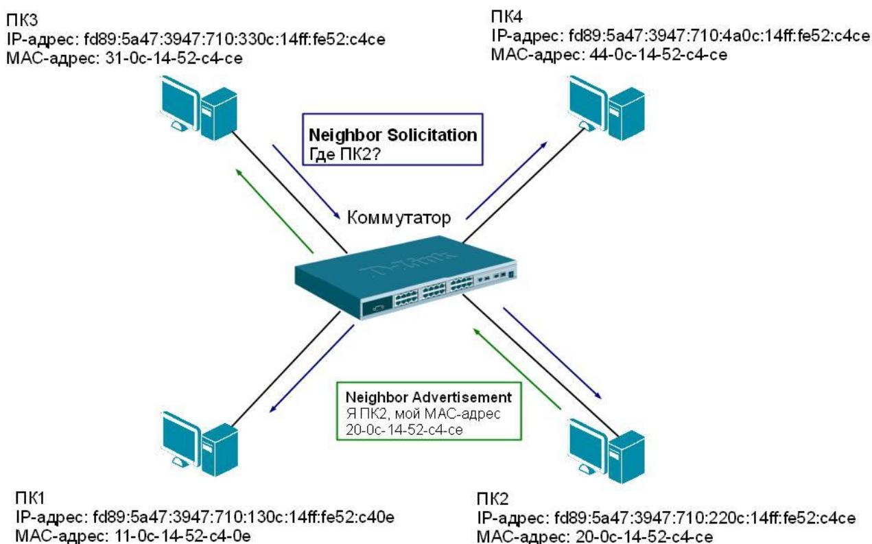
Рис. 5.35. Разрешение адресов с помощью протокола NDP
