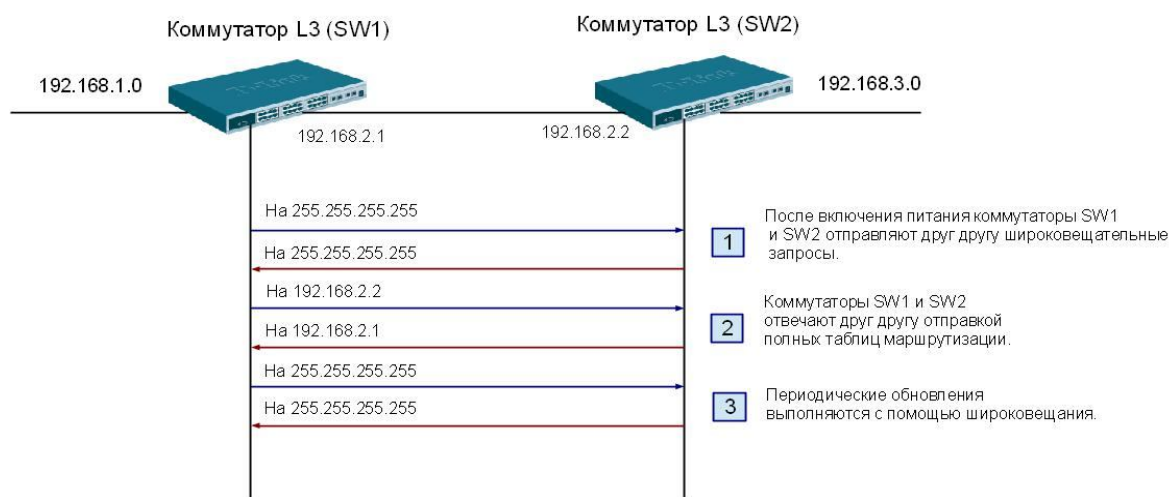
Рис. 5.52. Обмен RIP-сообщениями между коммутаторами 3-го уровня SW1 и SW2
