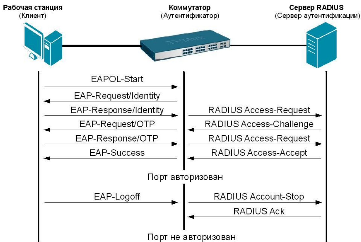
Рис. 7.15. Процесс аутентификации 802.1X
