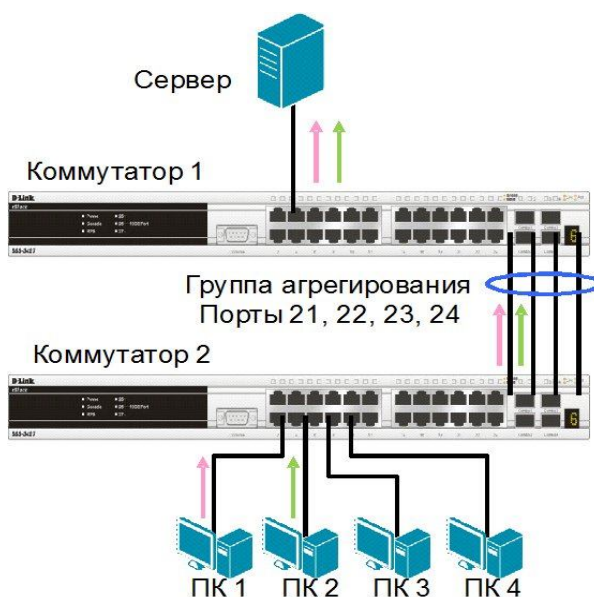
Рис. 4.29. Схема сети для настройки статического агрегирования канала
