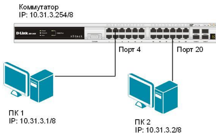
Рис. 7.23. Схема сети для настройки функций защиты ЦПУ
