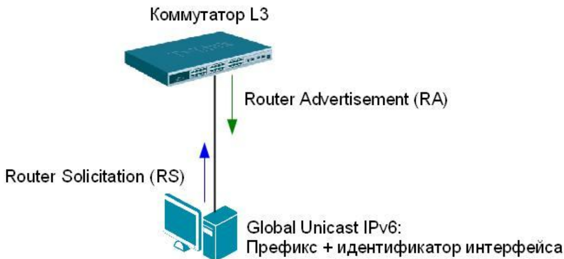
Рис. 5.32. Генерация Global Unicast-адреса при использовании механизма Stateless autoconfiguration
