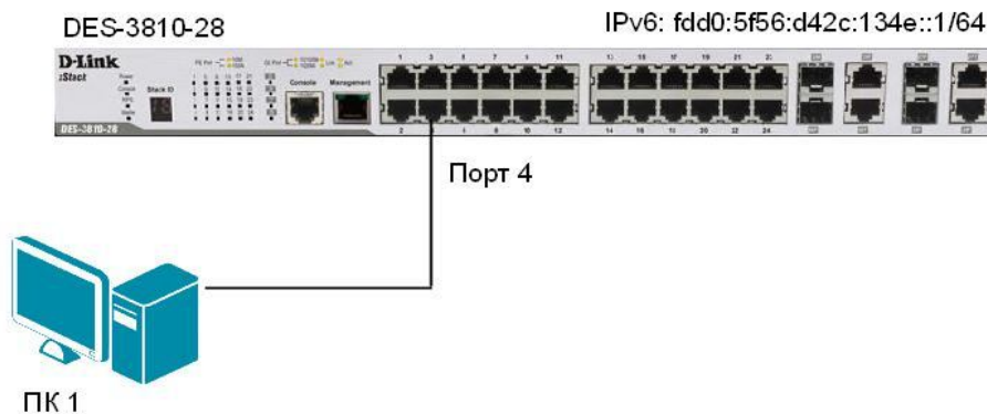
Рис. 5.33. Схема сети
