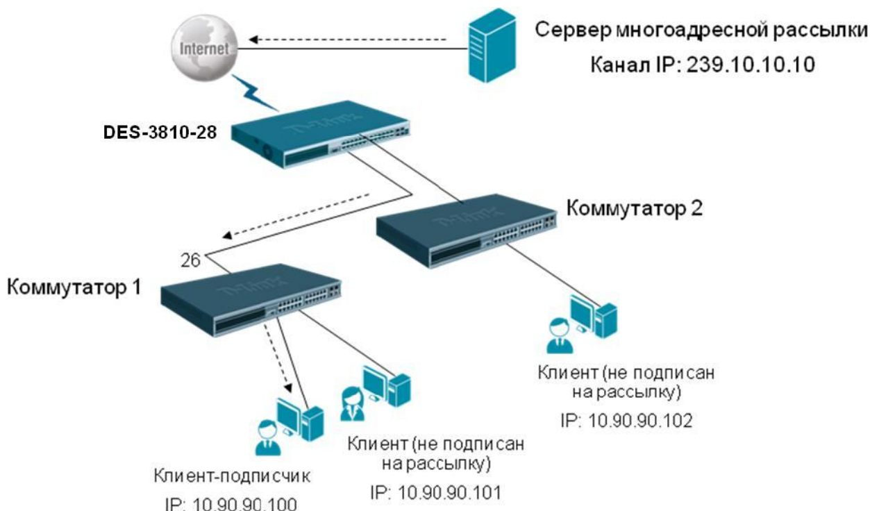
Рис. 8.6. Схема сети для настройки IGMP Snooping
