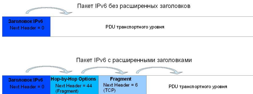
Рис. 5.20. Расширенные заголовки IPv6
