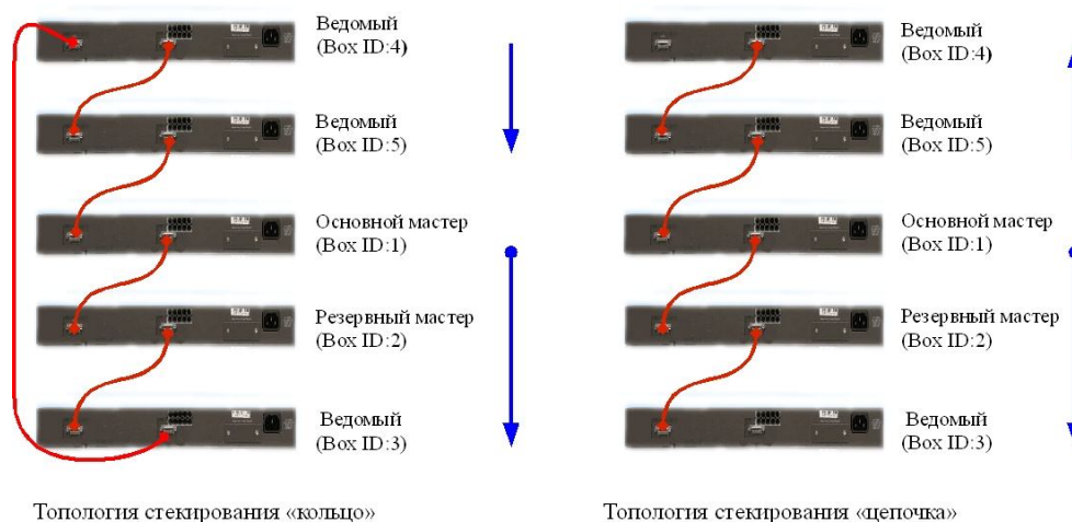
Рис. 9.5. Назначение порядковых номеров в автоматическом режиме
