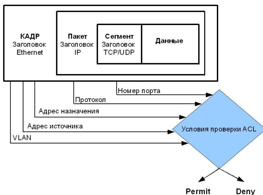
Рис. 7.1. Списки управления доступом (ACL)
