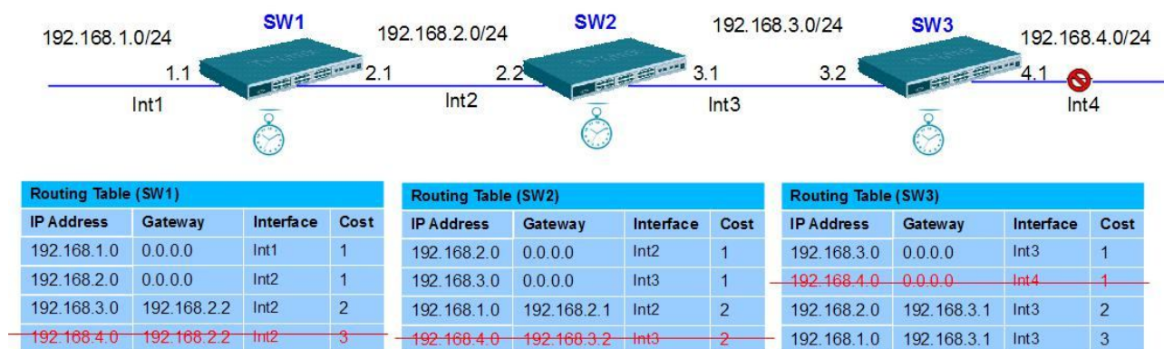
Рис. 5.51. Механизм установки таймера удержания
