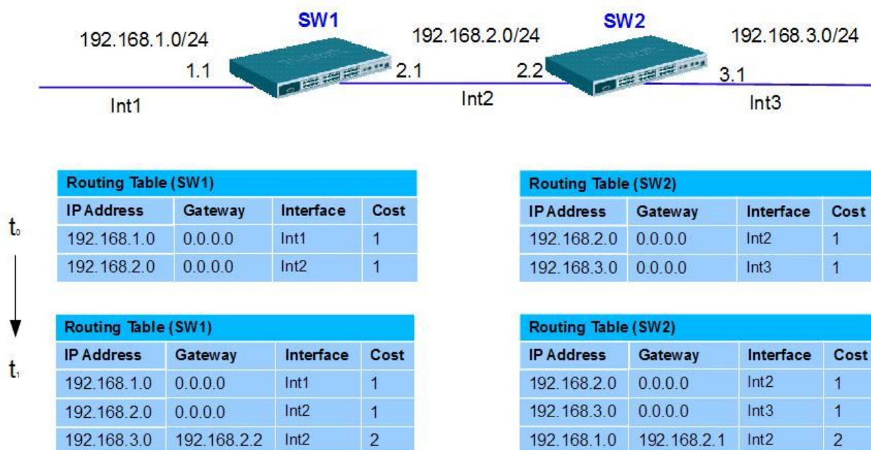
Рис. 5.46. Принцип работы дистанционно-векторного протокола
