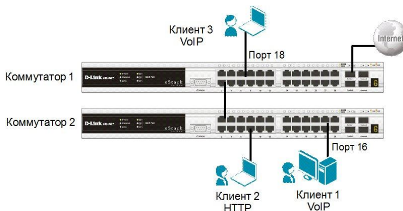
Рис. 6.11. Пример настройки QoS
