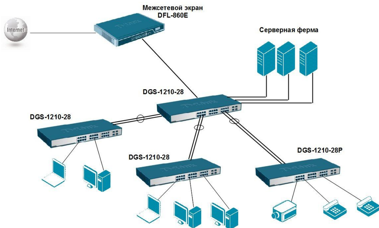
Рис. 10.5. Пример использования коммутаторов серии Smart в сетях SMB
