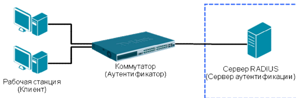
Рис. 7.13. Сервер аутентификации
