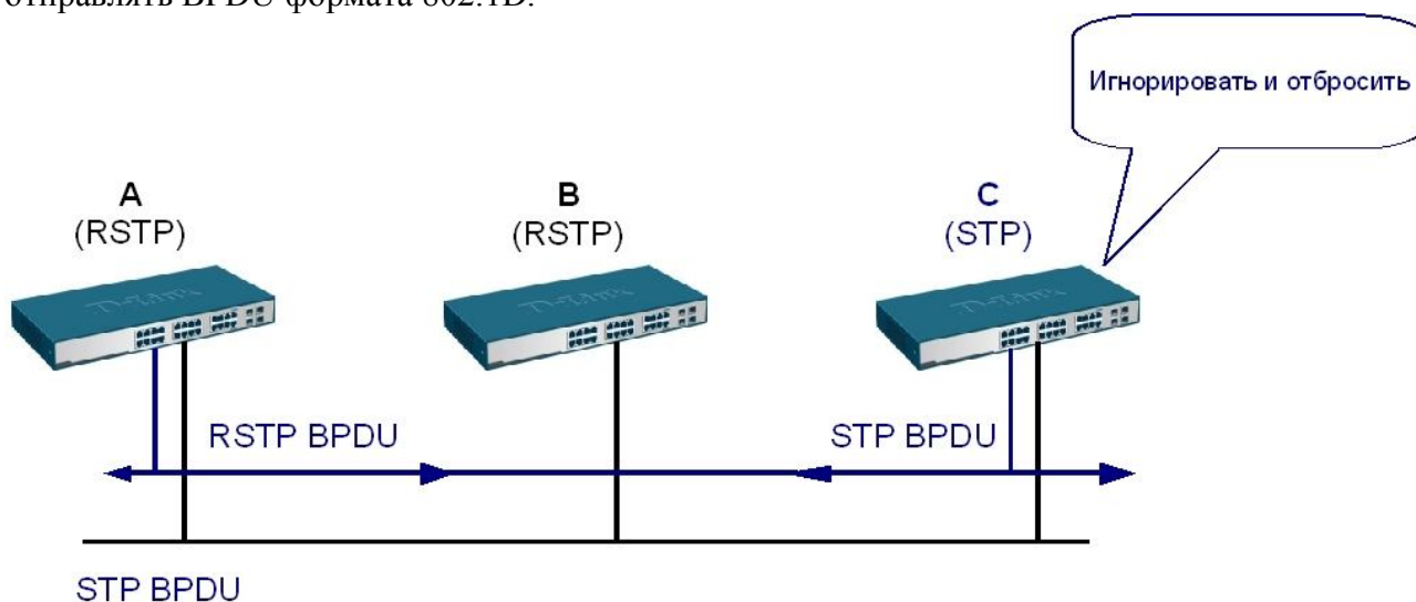
Рис. 4.16. Пример совместной работы коммутаторов с протоколами STP и RSTP
