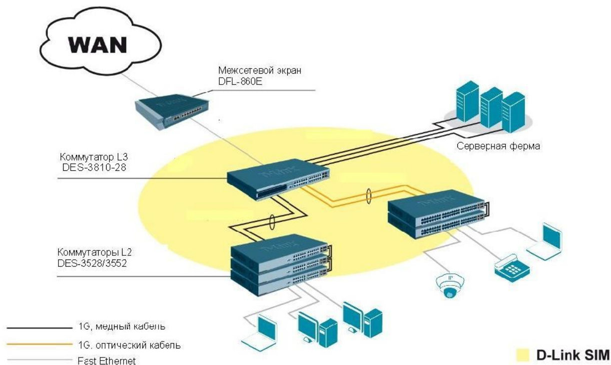
Рис. 9.7. Технология SIM
