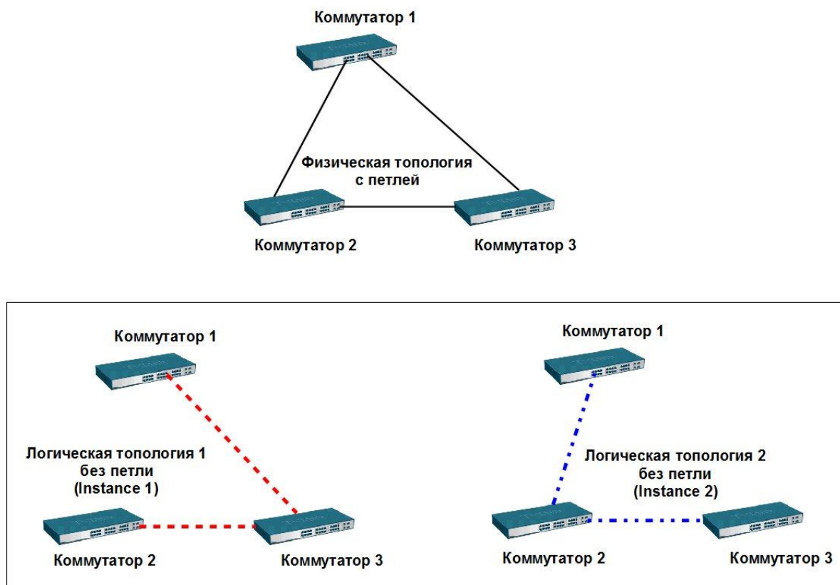
Рис. 4.18. Физическая и логическая топология региона MST
