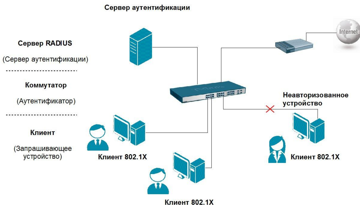
Рис. 7.11. Сеть с аутентификацией 802.1X
