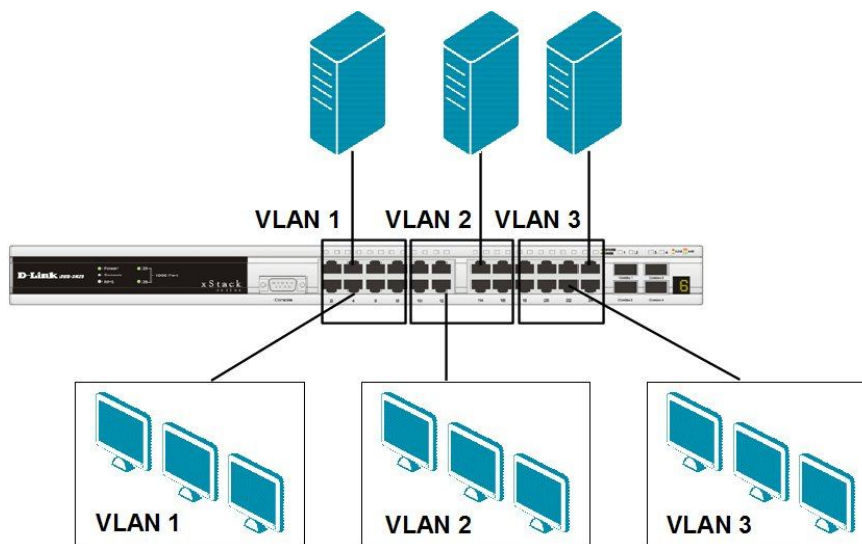
Рис. 3.3. VLAN на основе портов
