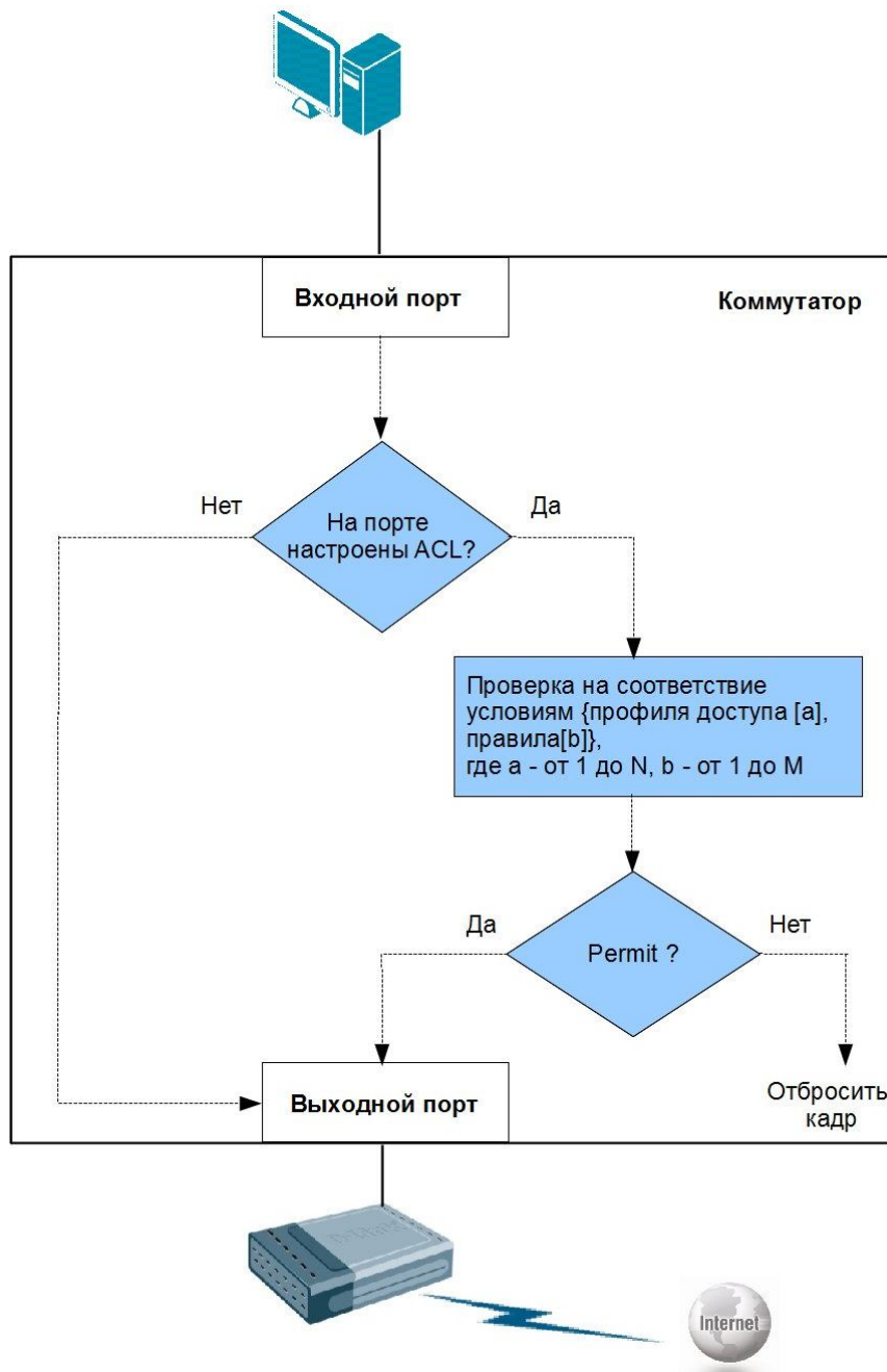
Рис. 7.2. Принцип работы ACL
