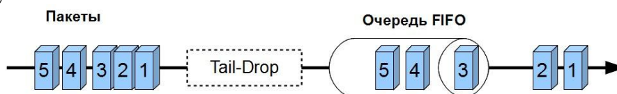
Рис. 6.5. Очередь FIFO
