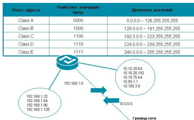
Рис. 5.55. Суммирование маршрутов на граничном маршрутизирующем устройстве
