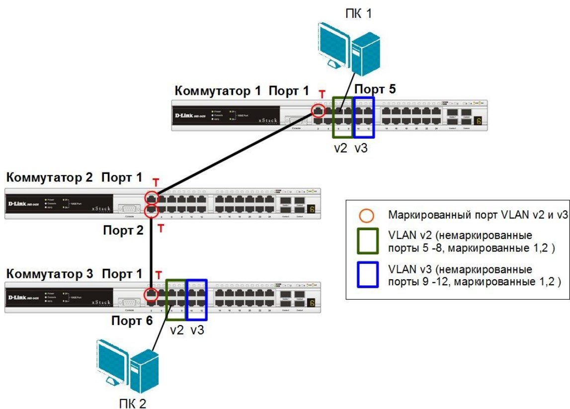
Рис. 3.14. Схема сети с двумя VLAN
