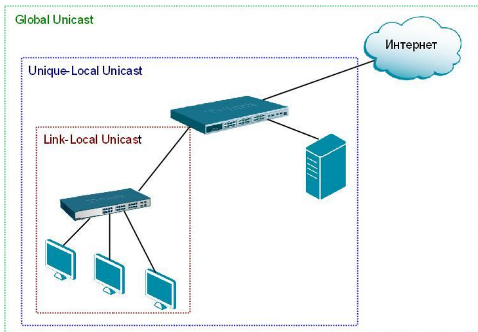
Рис. 5.22. Диапазон индивидуальных адресов IPv6
