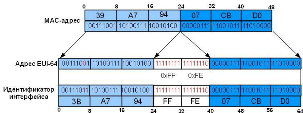
Рис. 5.31. Преобразование MAC-адреса в идентификатор интерфейса
