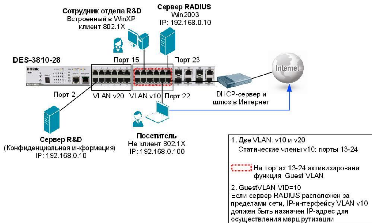
Рис. 7.21. Пример использования 802.1X Guest VLAN
