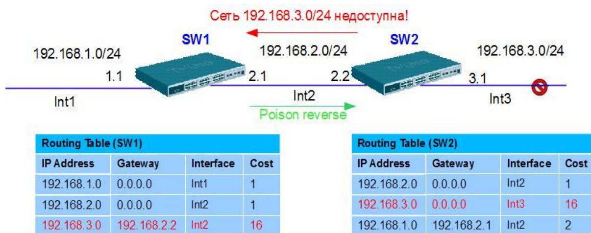
Рис. 5.50. Метод испорченного обратного маршрута
