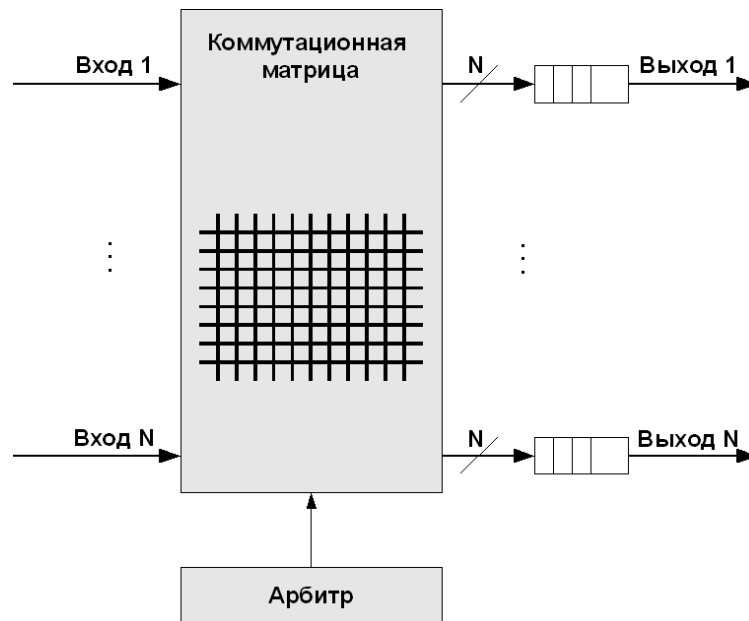
Рис. 1.19. Архитектура на основе коммутационной матрицы с выходными очередями
