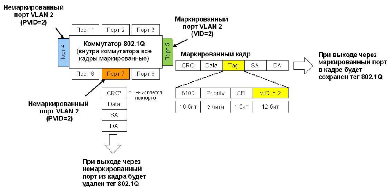
Рис. 3.13. Маркированный кадр, передаваемый через маркированный и немаркированный порты
