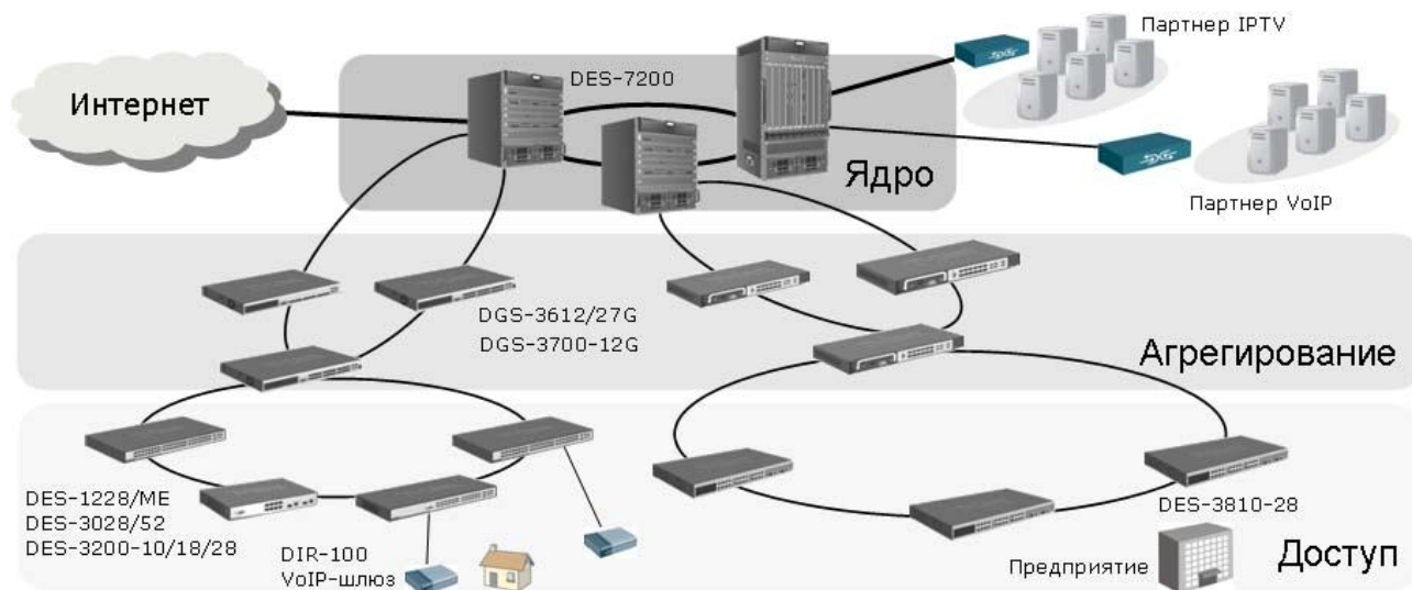
Рис. 10.13. Типовая схема применения коммутаторов D-Link
