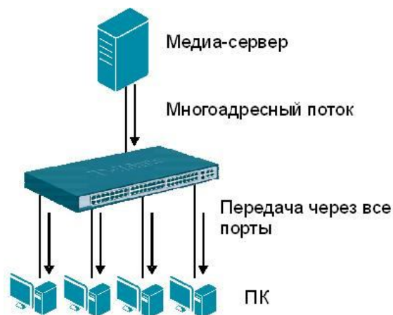
Рис. 8.3. Передача многоадресного трафика без поддержки управления им на коммутаторе
