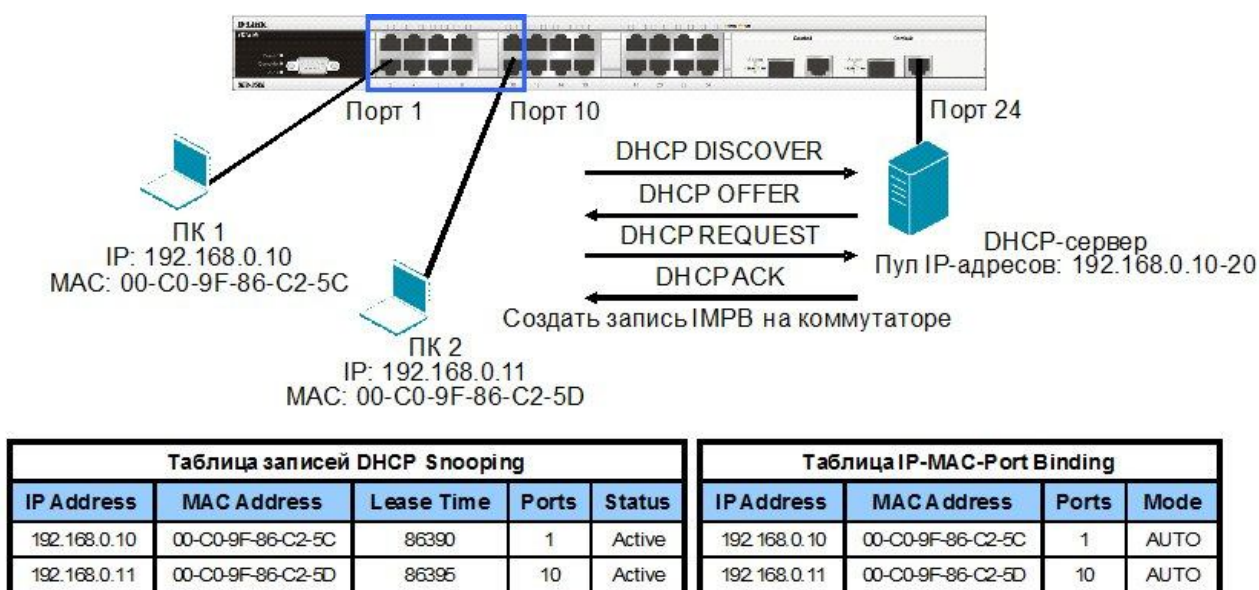
Рис. 7.10. Пример работы функции IP-MAC-Port Binding в режиме DHCP Snooping
