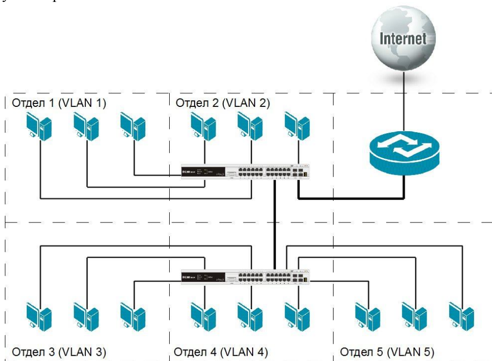
Рис. 3.2. Логическая группировка сетевых пользователей в VLAN
