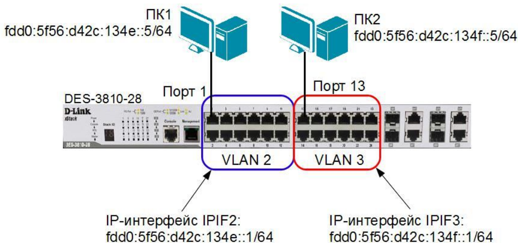
Рис. 5.43. Пример статической маршрутизации IPv6
