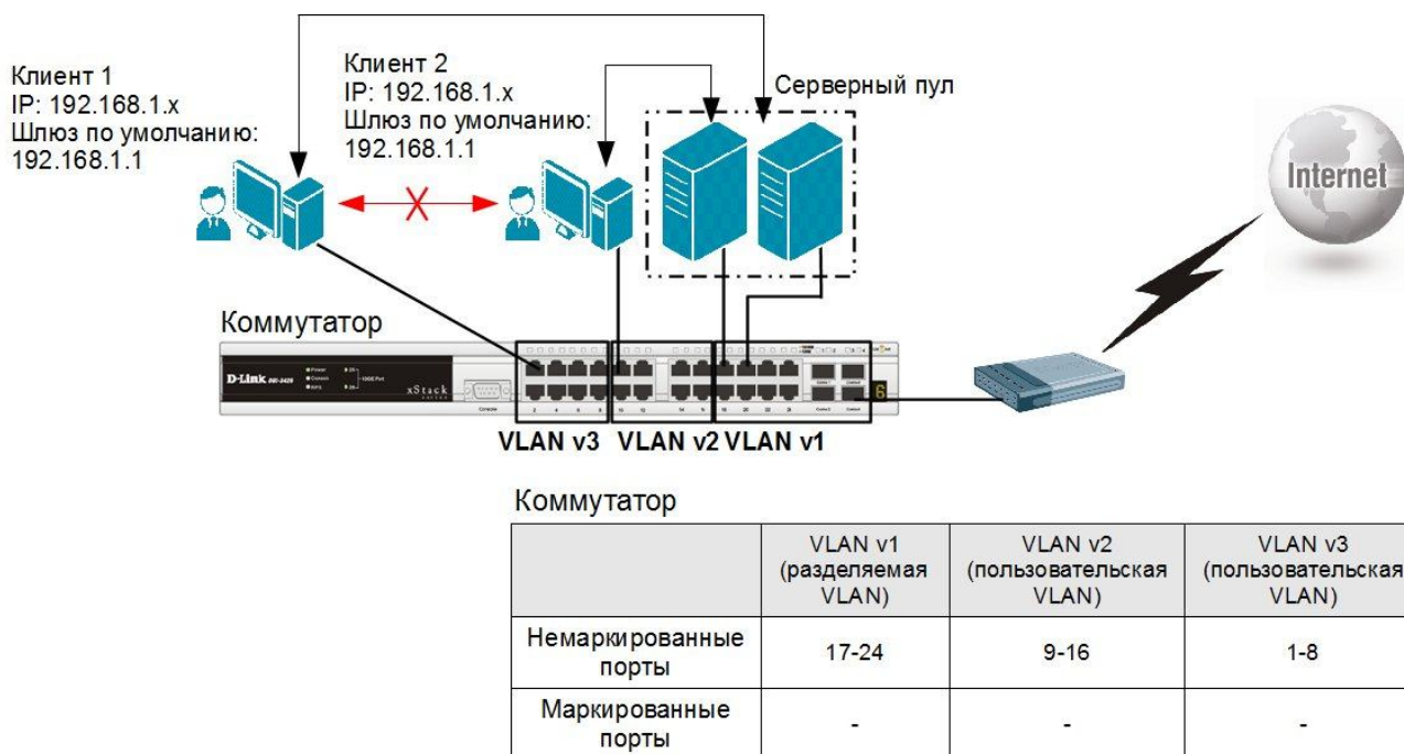
Рис. 3.24. Асимметричные VLAN в пределах одного коммутатора
