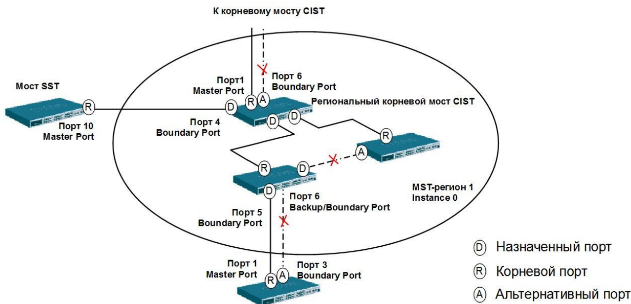
Рис. 4.22. Роли портов MSTP
