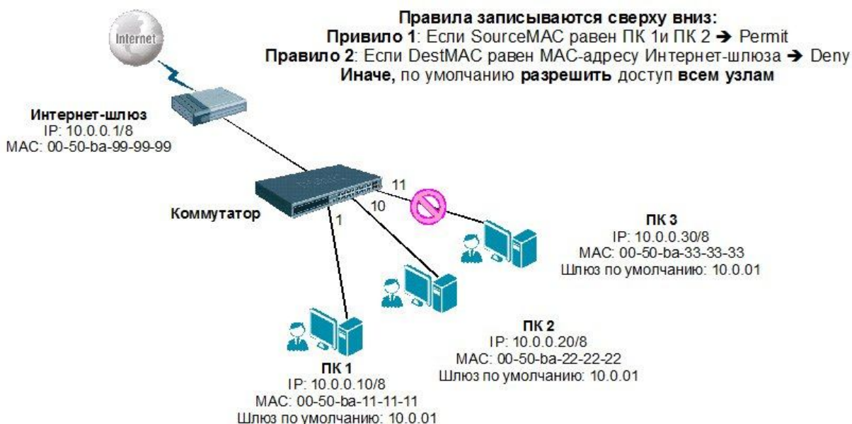
Рис. 7.4. Пример ACL для профиля Ethernet
