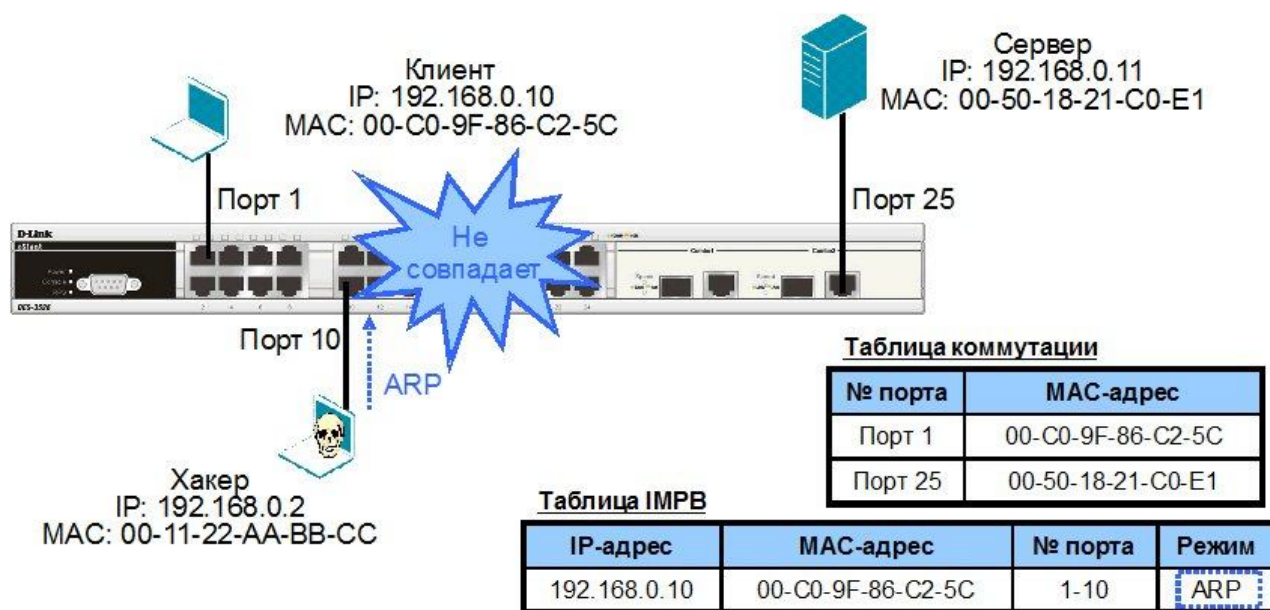
Рис. 7.9. Пример работы функции IP-MAC-Port Binding в режиме ARP
