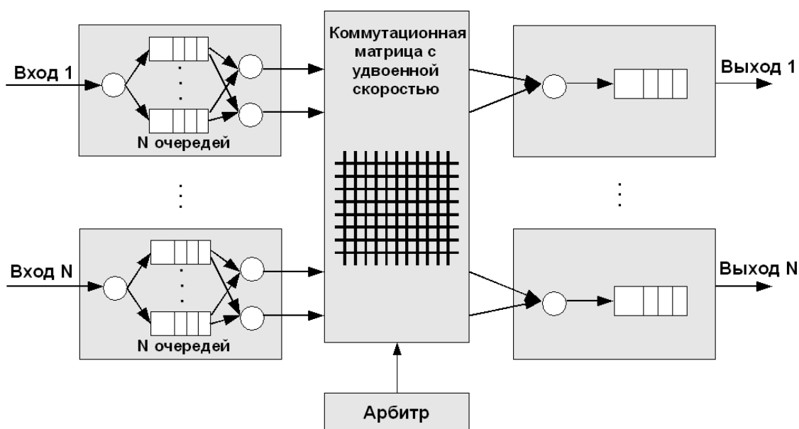
Рис. 1.21. Архитектура на основе коммутационной матрицы с CIOQ
