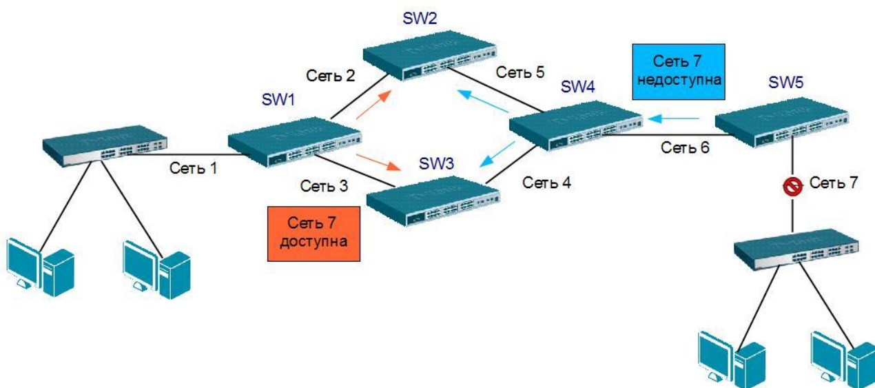
Рис. 5.47. Проблемы при работе дистанционно-векторного алгоритма маршрутизации
