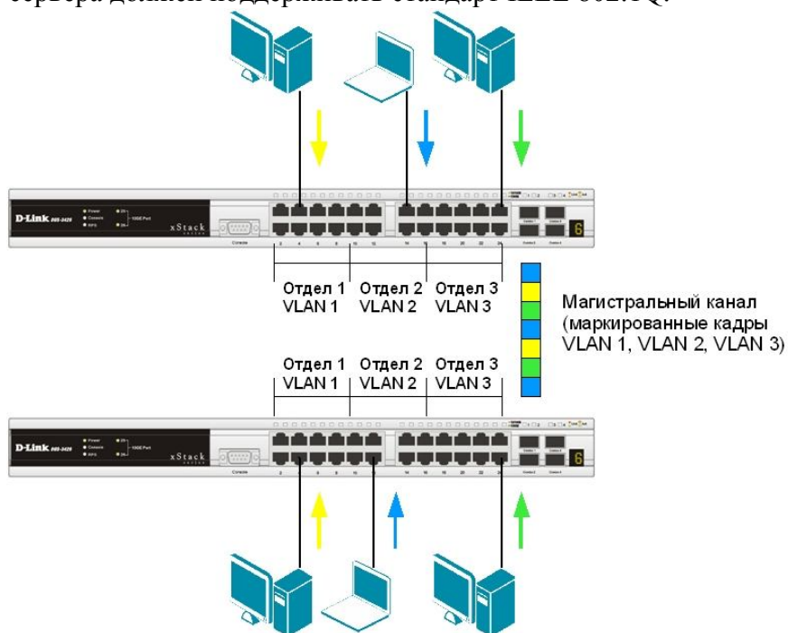
Рис. 3.5. Передача кадров нескольких VLAN по магистральному каналу связи
