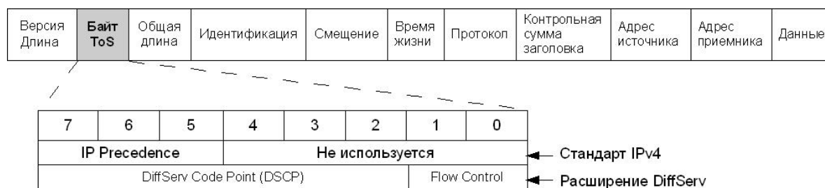
Рис. 6.2. Байт ToS заголовка IPv4
