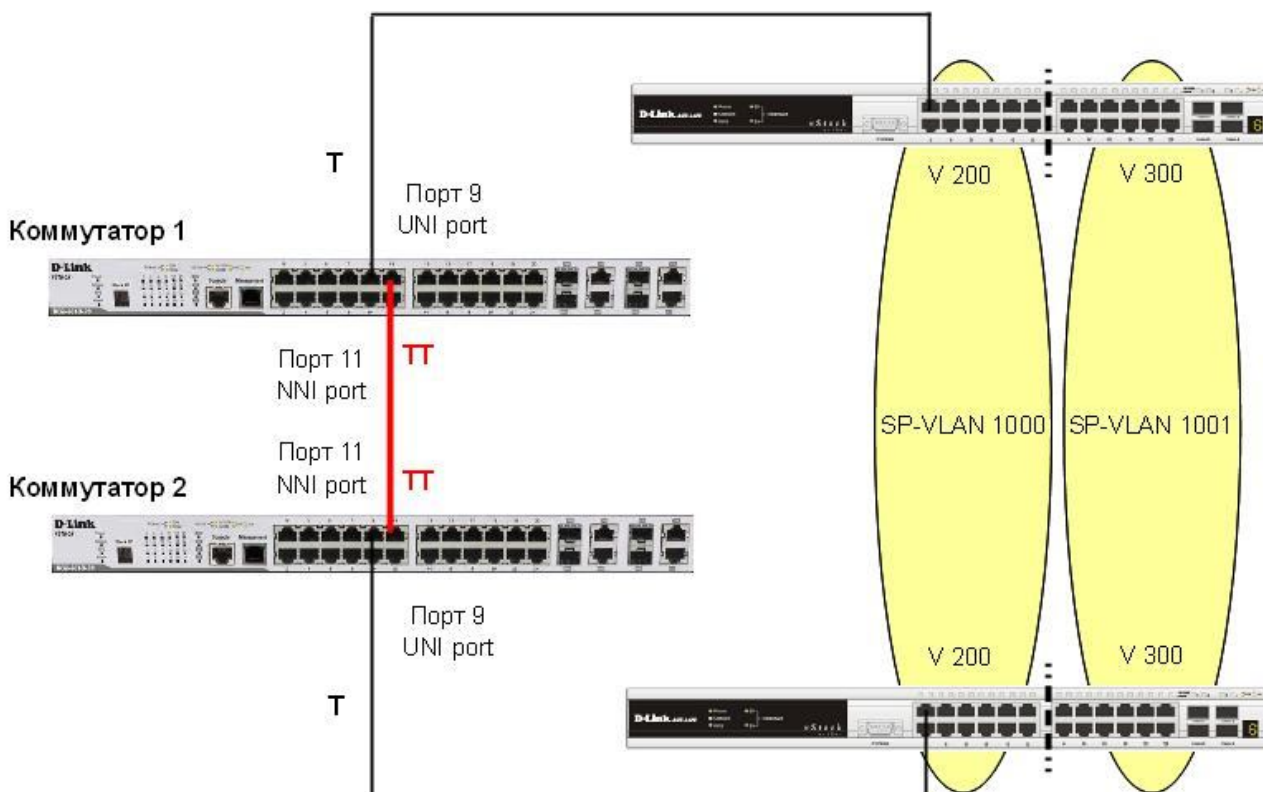
Рис. 3.21. Схема подключения клиентских VLAN к пограничным коммутаторам сети провайдера услуг
