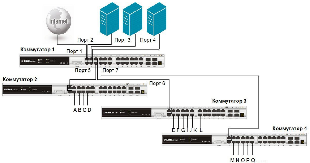
Рис. 3.26. Иерархическая структура Traffic Segmentation
