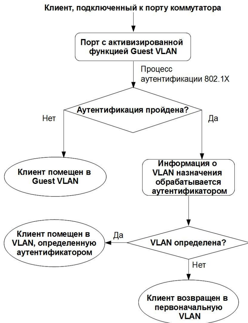
Рис. 7.19. Процесс аутентификации с использованием Guest VLAN
