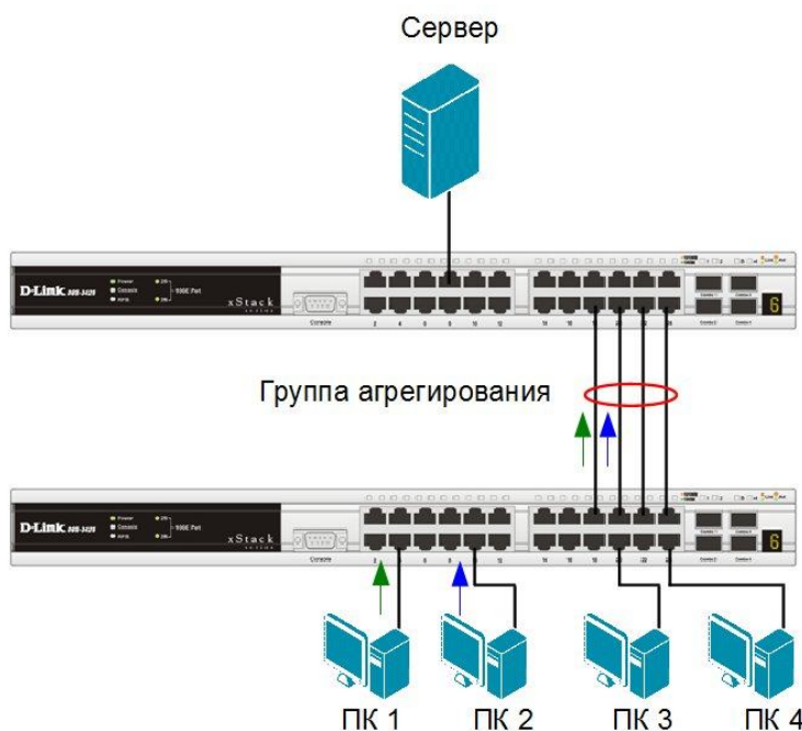
Рис. 4.27. Пример агрегированного канала связи между коммутаторами
