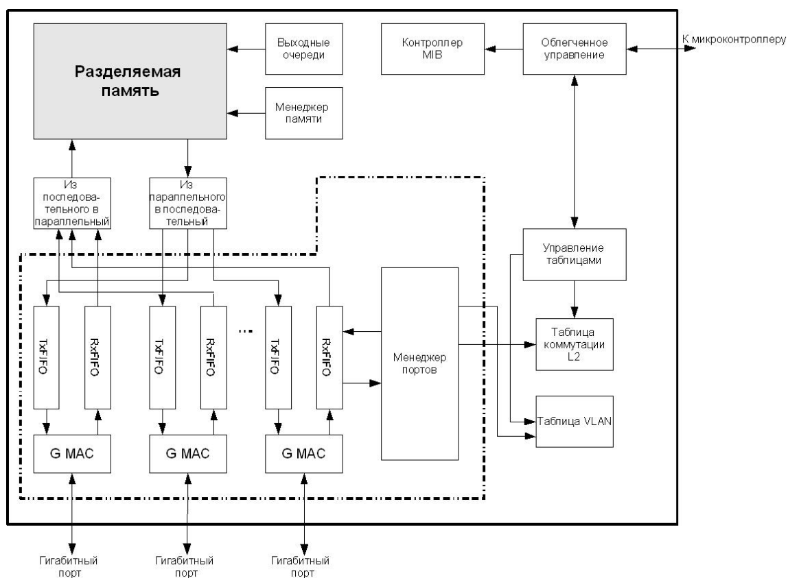
Рис. 1.16. Архитектура с разделяемой памятью
