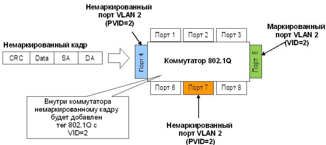
Рис. 3.10. Входящий немаркированный кадр
