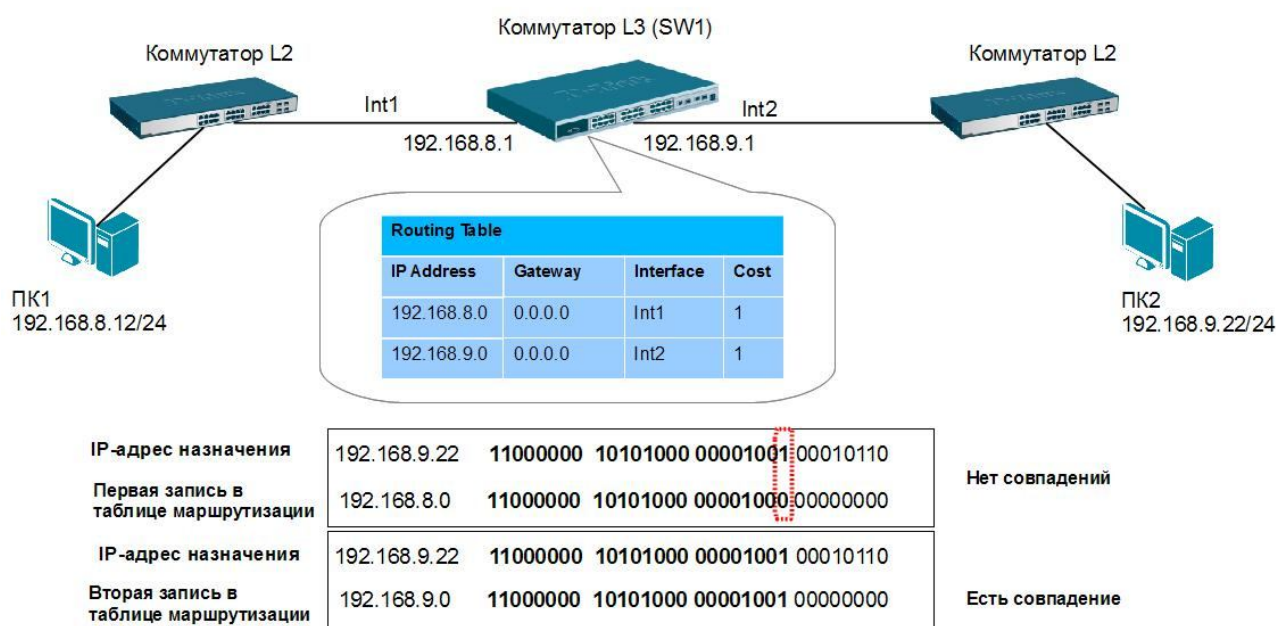
Рис. 5.41. Процесс поиска маршрута в таблице маршрутизации
