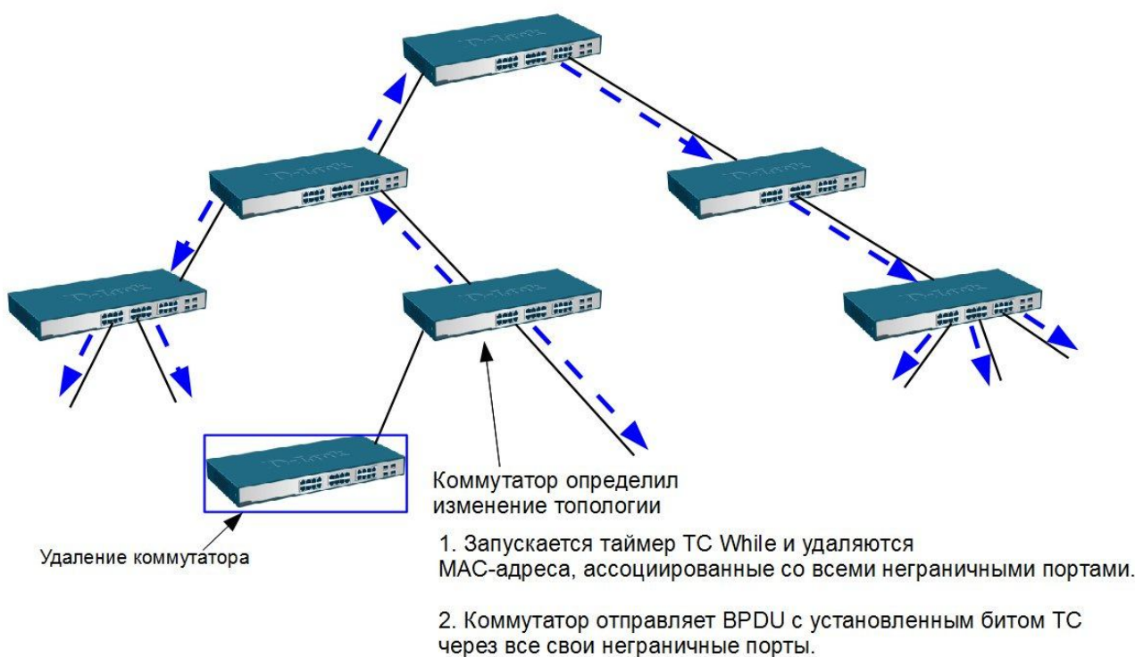
Рис. 4.15. Новый механизм изменения топологии
