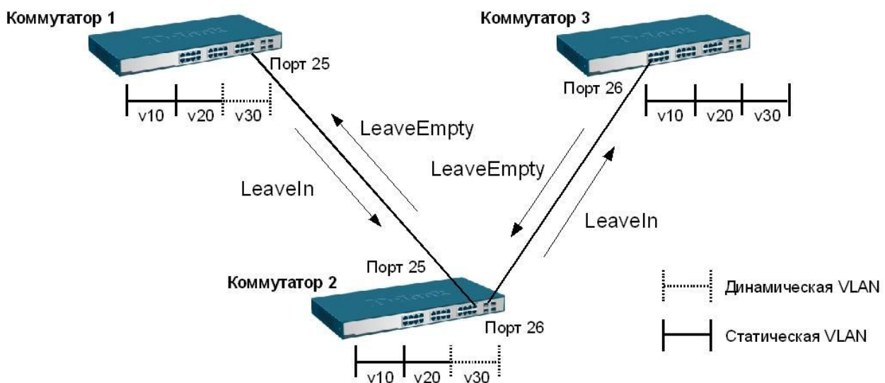
Рис. 3.16. Процесс распространения информации об удалении VLAN по сети
