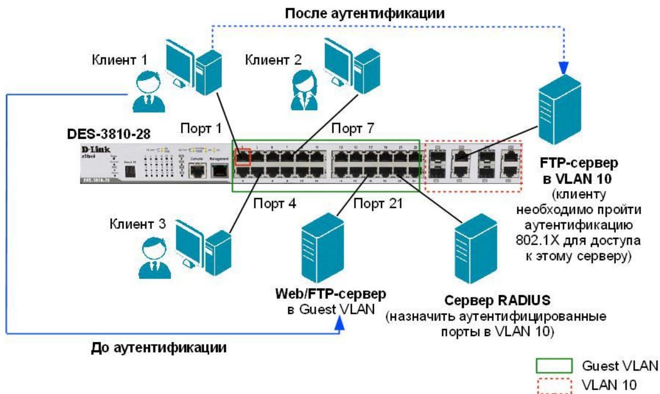
Рис. 7.20. Ресурсы доступные клиенту до и после аутентификации 802.1X при использовании Guest VLAN
