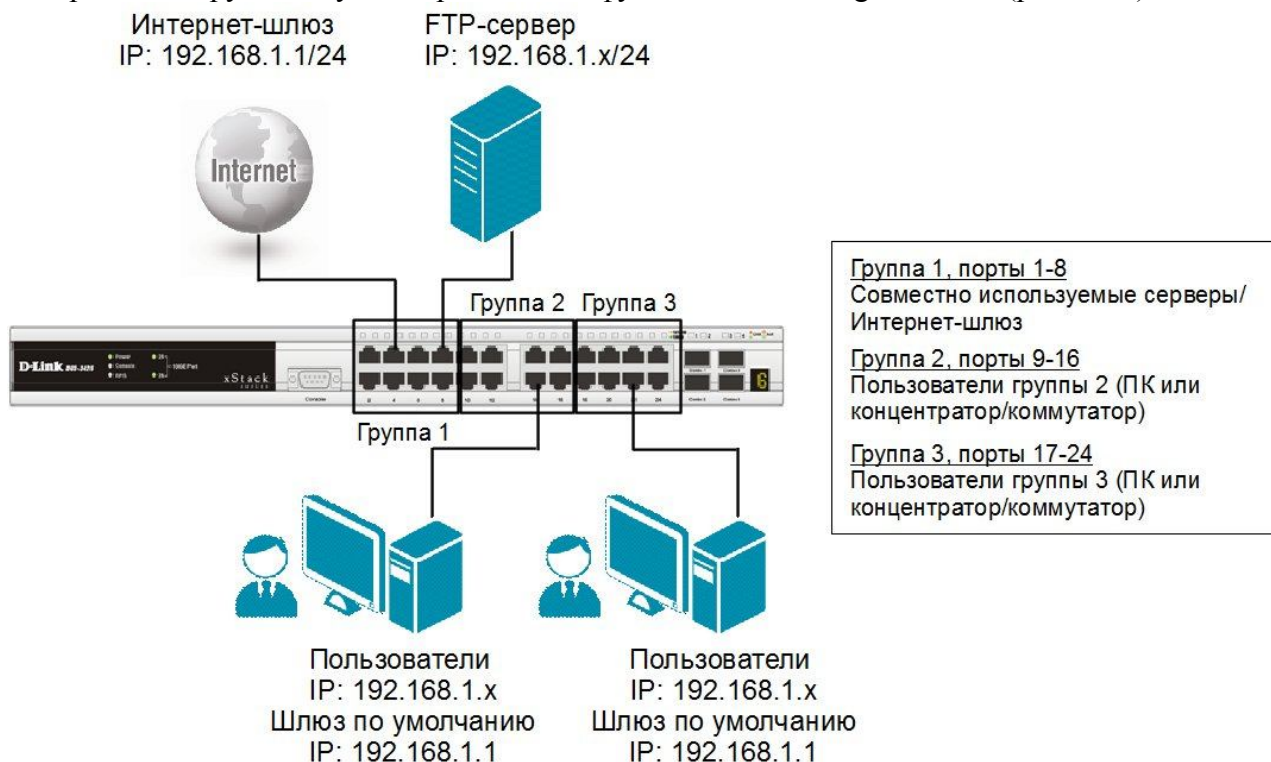
Рис. 3.25. Пример использования функции Traffic Segmentation
