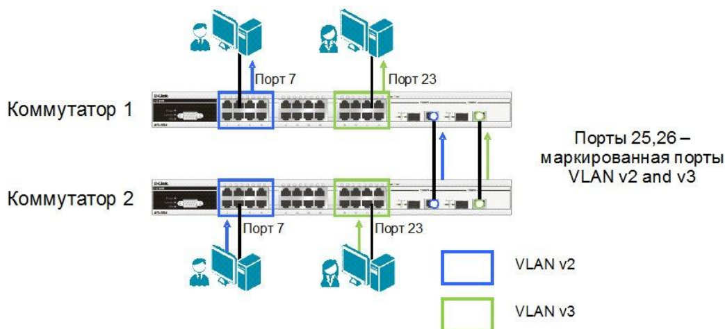
Рис. 4.25. Балансировка нагрузки с помощью MSTP
