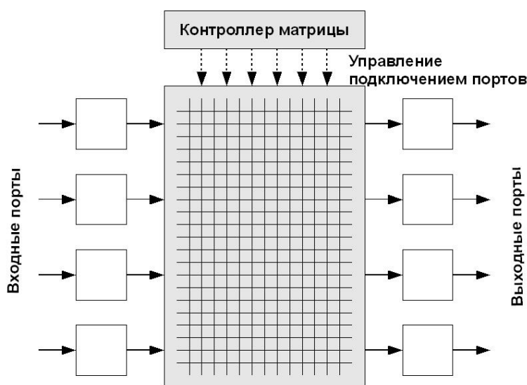
Рис. 1.17. Архитектура на основе коммутационной матрицы
