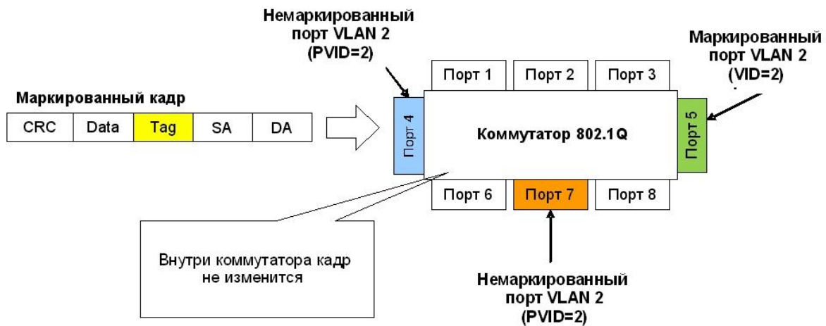
Рис. 3.12. Входящий маркированный кадр
