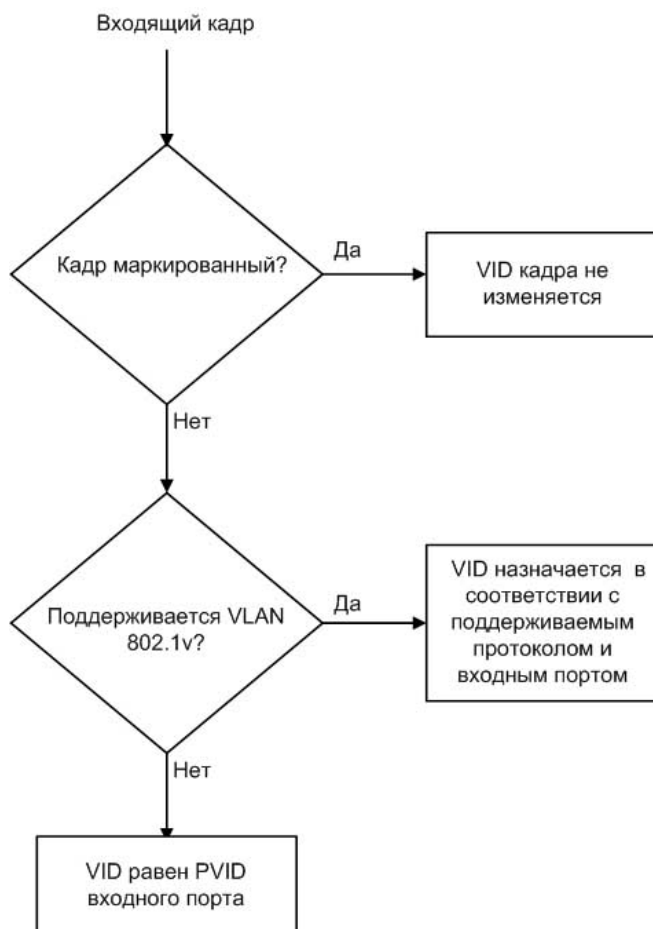
Рис. 3.22. Правила классификации входящих кадров
