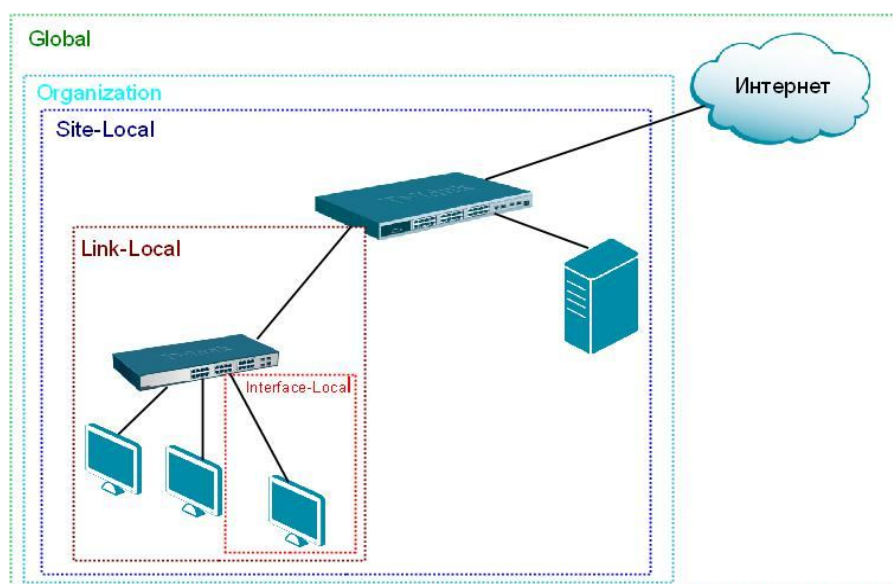
Рис. 5.27. Области действия многоадресных адресов IPv6
