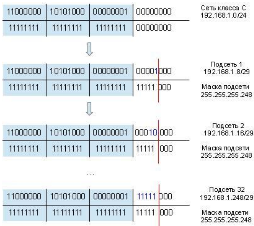
Рис. 5.16. Пример разбиения сети 192.168.1.0/24 на подсети
