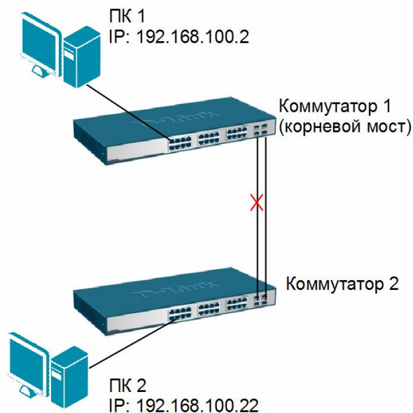
Рис. 4.17. Схема сети для настройки RSTP
