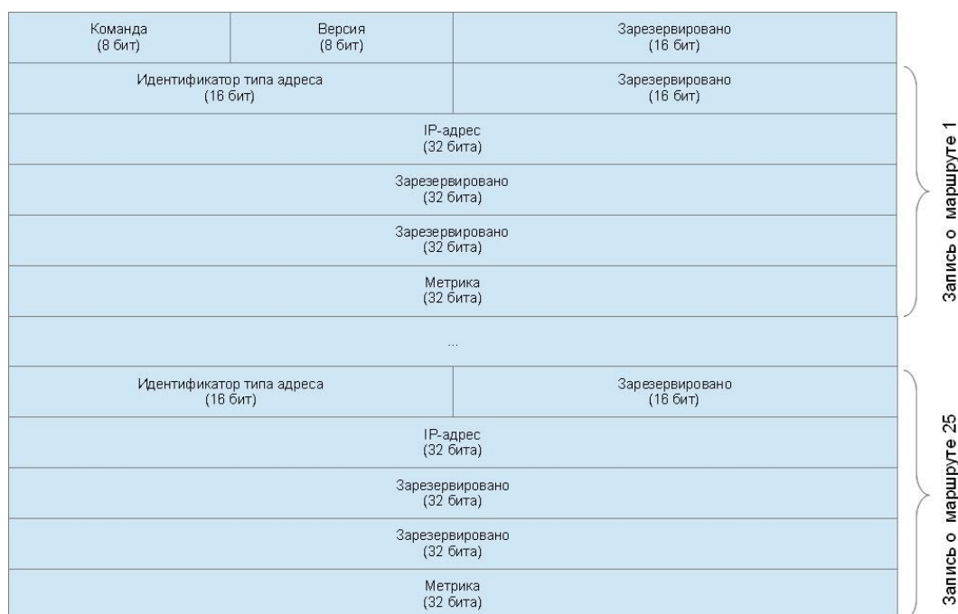
Рис. 5.53. Формат сообщения протокола RIPv1
