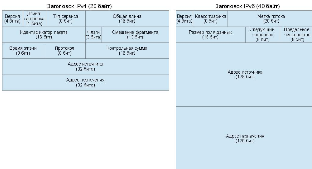
Рис. 5.19. Сравнение форматов заголовка IPv4 и IPv6
