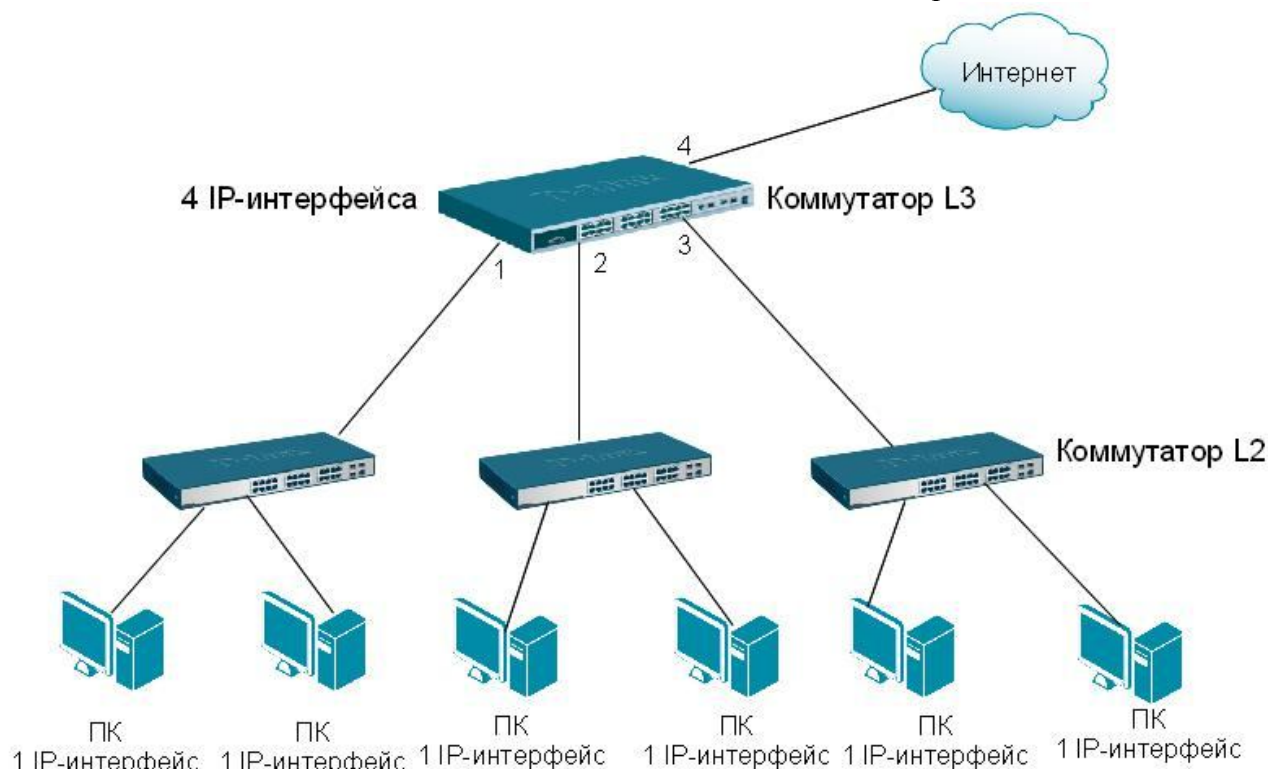
Рис. 5.3. IP-интерфейсы устройств
