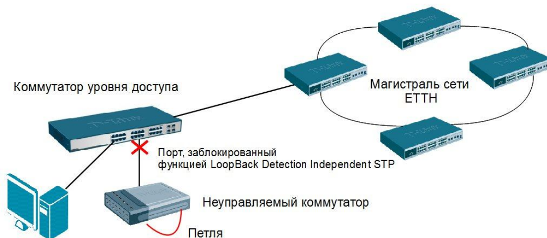
Рис. 4.26. Пример работы функции LoopBack Detection Independent STP
