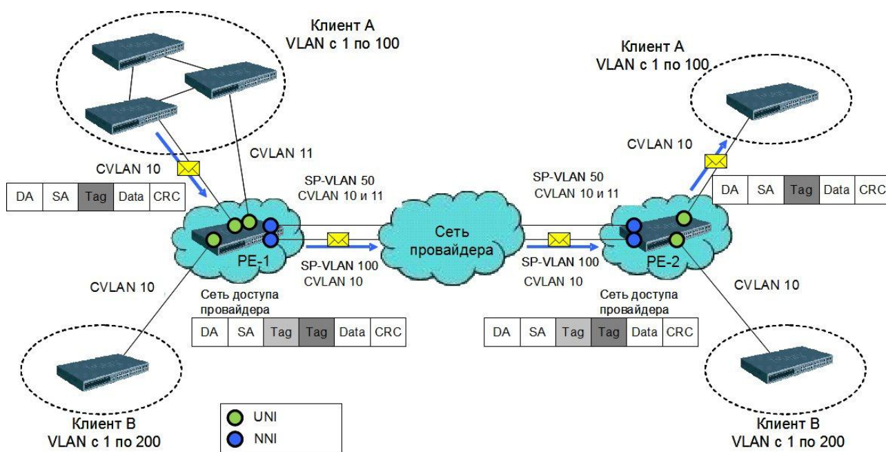
Рис. 3.19. Базовая архитектура сети провайдера с применением функции Port-based Q-in-Q
