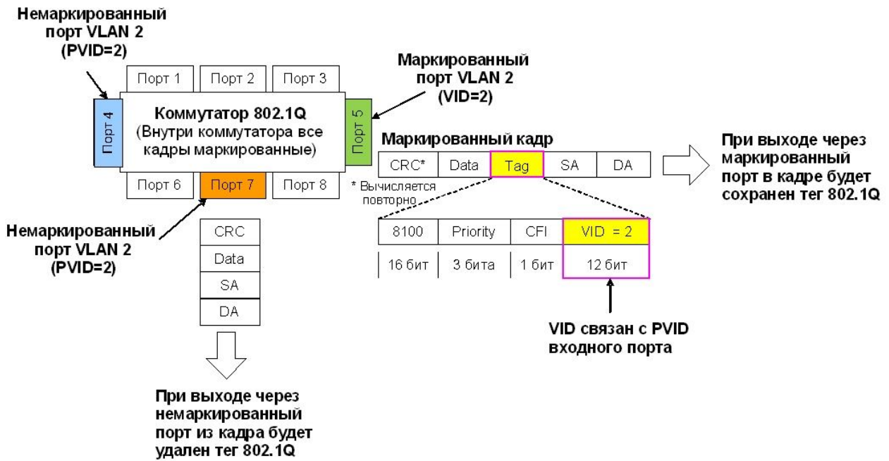
Рис. 3.11. Немаркированный кадр, передаваемый через маркированный и немаркированный порты
