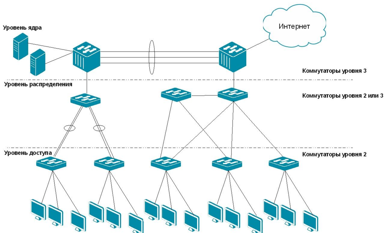
Рис. 1.24. Трехуровневая модель сети
