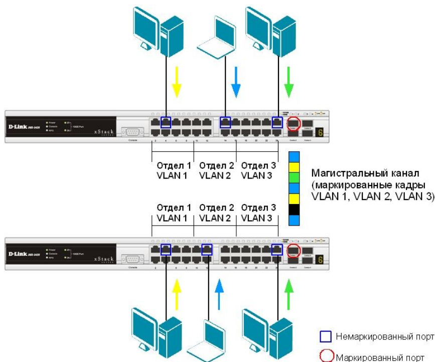
Рис. 3.6. Маркированные и немаркированные порты VLAN
