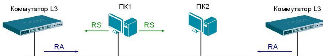
Рис. 5.38. Обнаружение локального коммутатора L3
