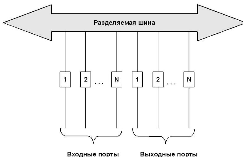
Рис. 1.15. Архитектура с разделяемой шиной
