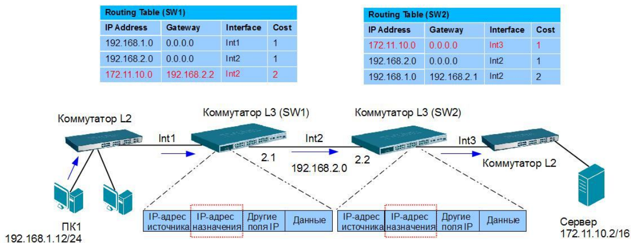
Рис. 5.40. Процесс обработки пакета маршрутизаторами
