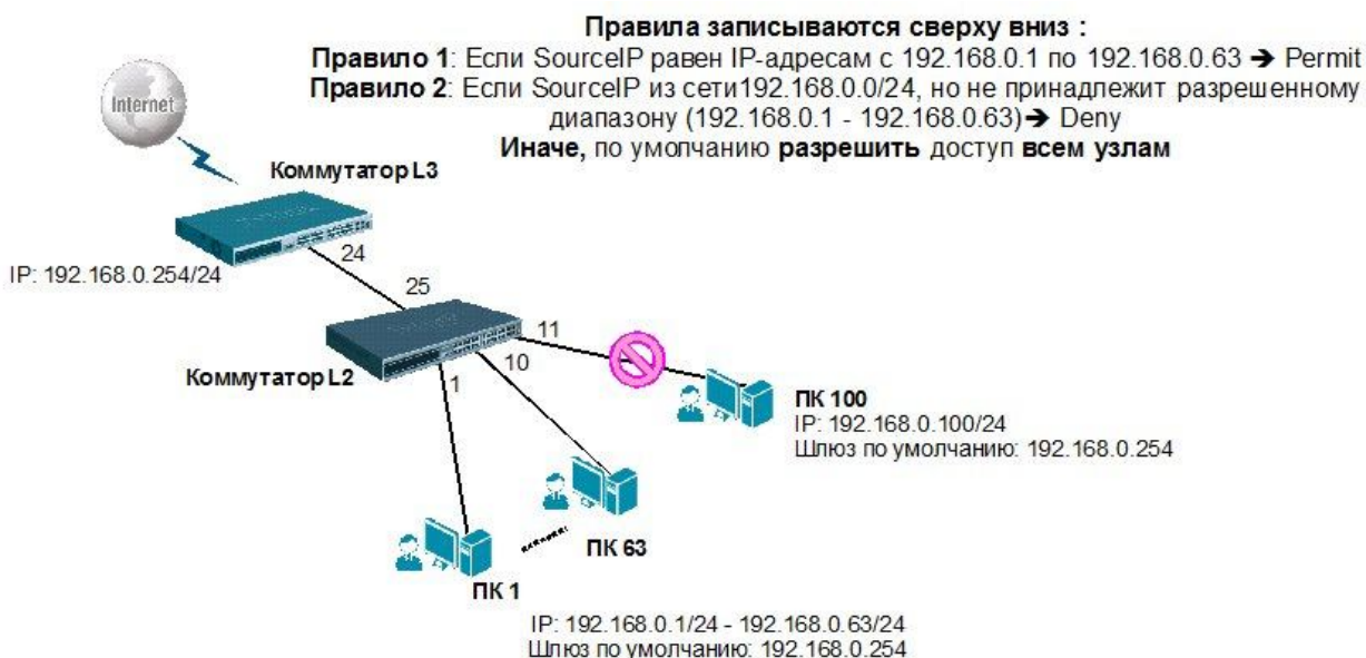
Рис. 7.5. Пример ACL для профиля IP
