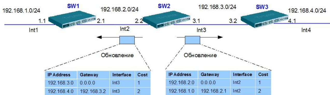
Рис. 5.49. Механизм расщепления горизонта
