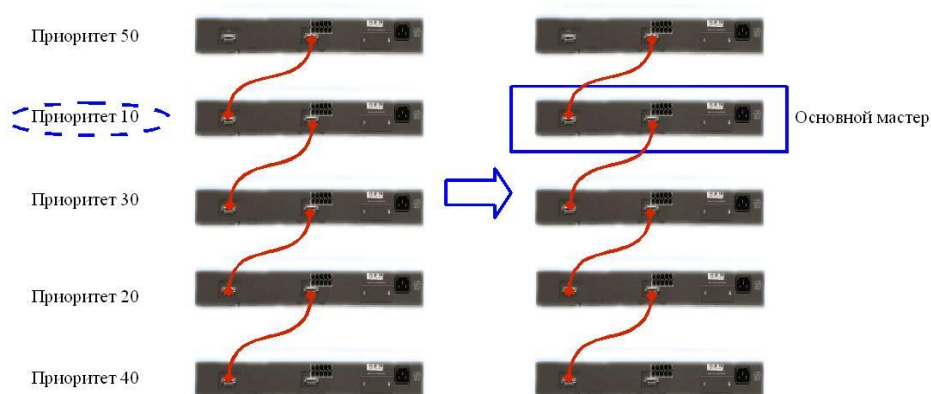
Рис. 9.3. Процесс выбора основного мастера на основании приоритетов
