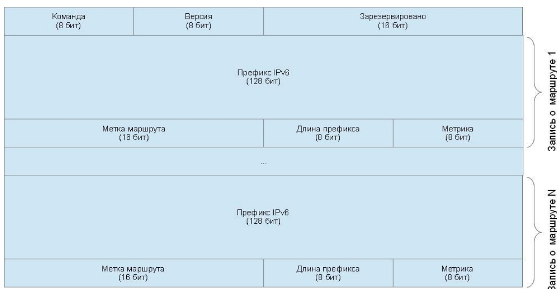
Рис. 5.58. Формат сообщения протокола RIPng
