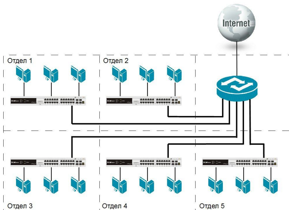
Рис. 3.1. Физическая сегментация сети
