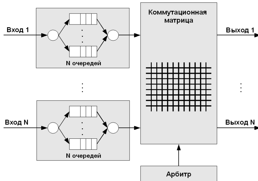
Рис. 1.20. Архитектура на основе коммутационной матрицы с виртуальными очередями
