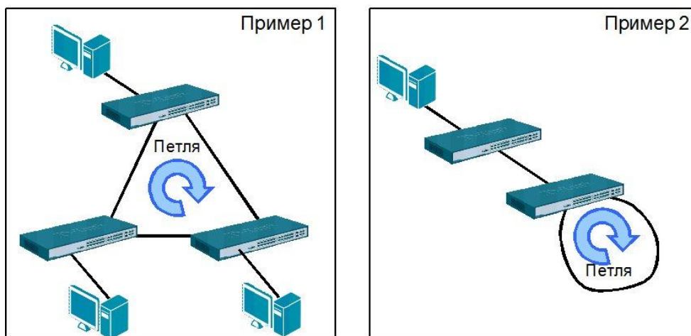
Рис. 4.1. Примеры петель между коммутаторами
