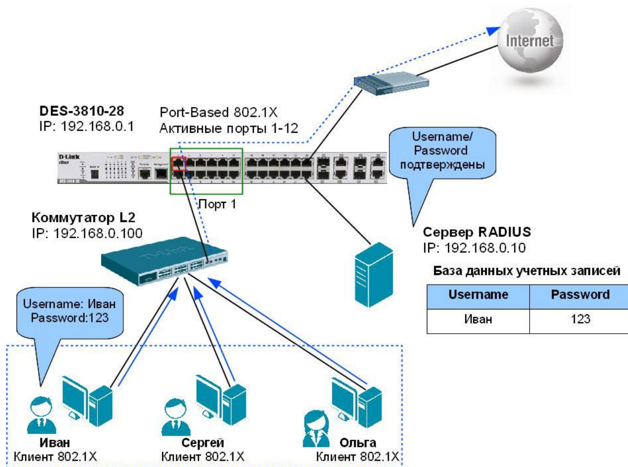
Рис. 7.16. Аутентификация 802.1X на основе портов
